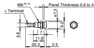
ø6 IPL1-67
