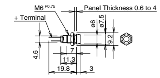
ø6 IPL1-69
