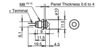
ø6 IPL1-69
