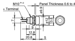
ø6 IPL1-67
