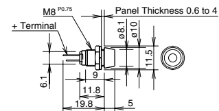
ø8 IPL1-89
