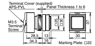
ø22 EB3P-LUW1B
